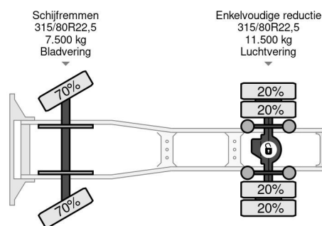
MAN 19.403 F2000 SLEEPERCAB (EURO 2 / ZF16 M... 4x2
